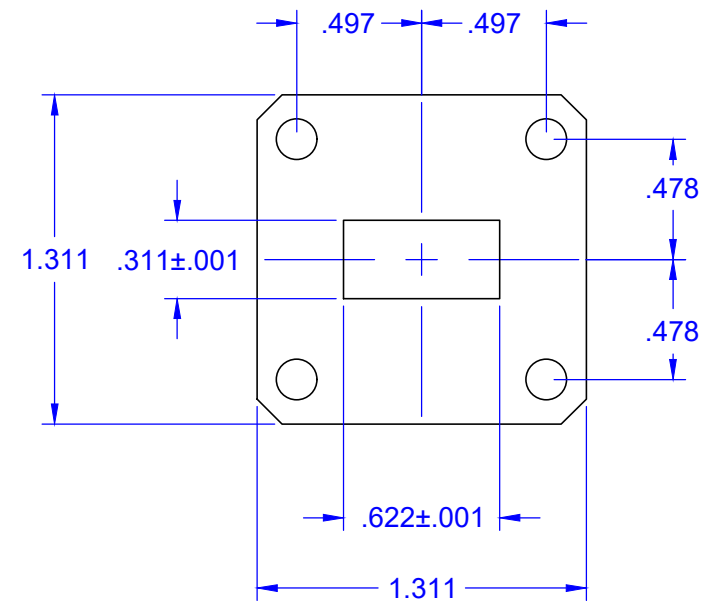
UG-419 FLANGE
