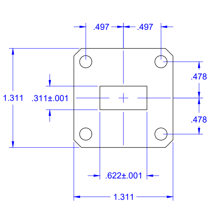
UG-419 FLANGE
